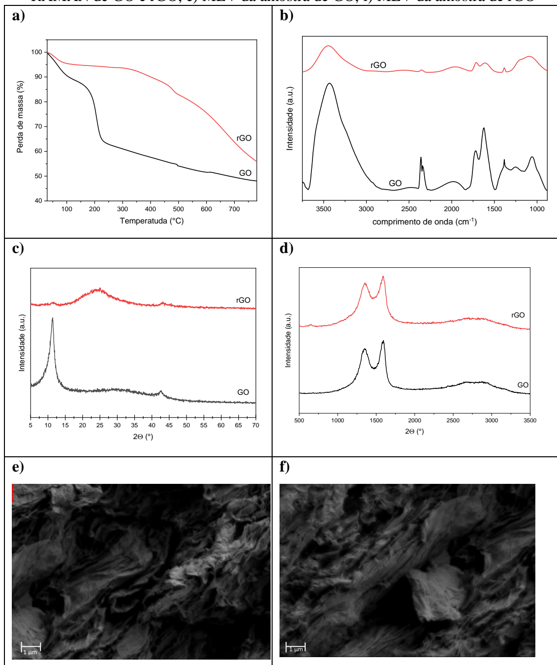
Figura 2: Caracterização das amostras de GO e rGO, a) Termograma de GO e rGO, b) Espectros de FTIR de GO e rGO, c) Difratograma de GO e rGO, d) Espectros de RAMAN de GO e rGO, e) MEV da amostra de GO, f) MEV da amostra de rGO
